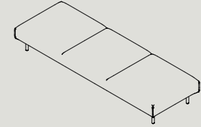
HO3-LOFT W 2490 D 830 H 410 W 98" D 32.7" H 16.2"
