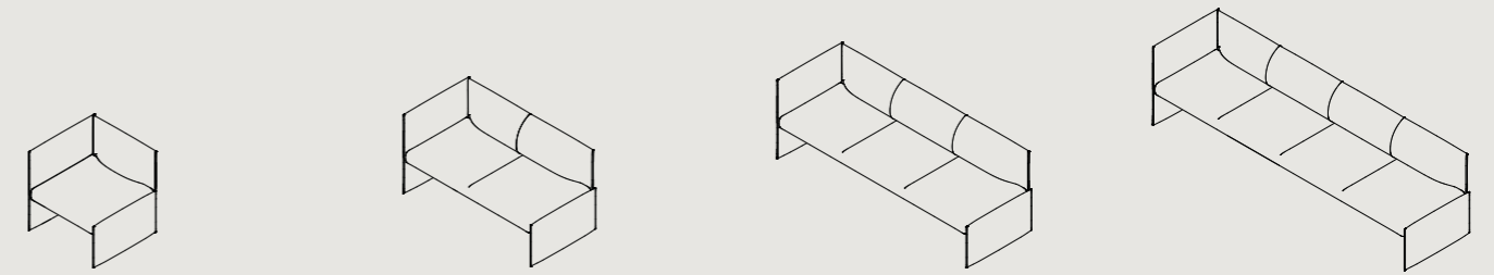
DA1-R/L* W 790 D 740 H 740 S 440 DA2-R/L* W 1450 D 740 H 740 S 440 DA3-R/L* W 2110 D 740 H 740 S 440 DA4-R/L* W 2770 D 740 H 740 S 440
