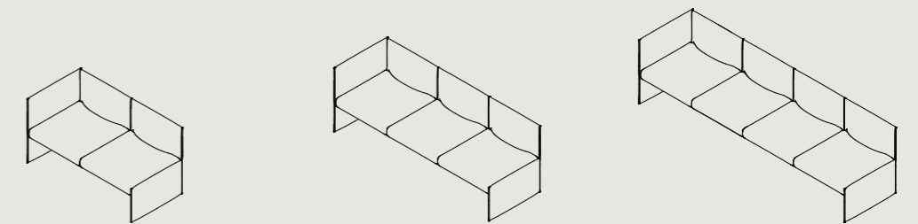
DA2-IND-R/L* W 1450 D 740 H 740 S 440 DA3-IND-R/L* W 2110 D 740 H 740 S 440 DA4-IND-R/L* W 2770 D 740 H 740 S 440
