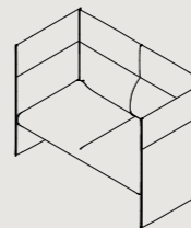
DML2 W 1450 D 740 H 1020 S 440
