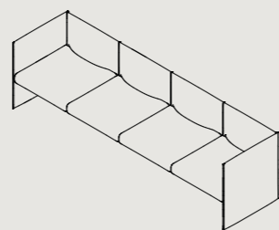
DL4-IND W 2770 D 740 H 740 S 440
