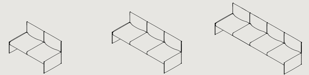
DB2-IND W 1450 D 740 H 740 S 440 DB3-IND W 2110 D 740 H 740 S 440 DB4-IND W 2770 D 740 H 740 S 440
