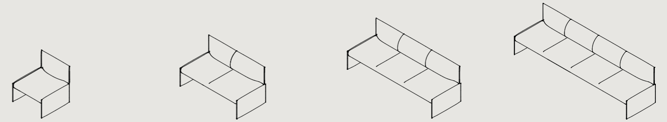
DB1 W 790 D 740 H 740 S 440 DB2 W 1450 D 740 H 740 S 440 DB3 W 2110 D 740 H 740 S 440 DB4 W 2770 D 740 H 740 S 440
