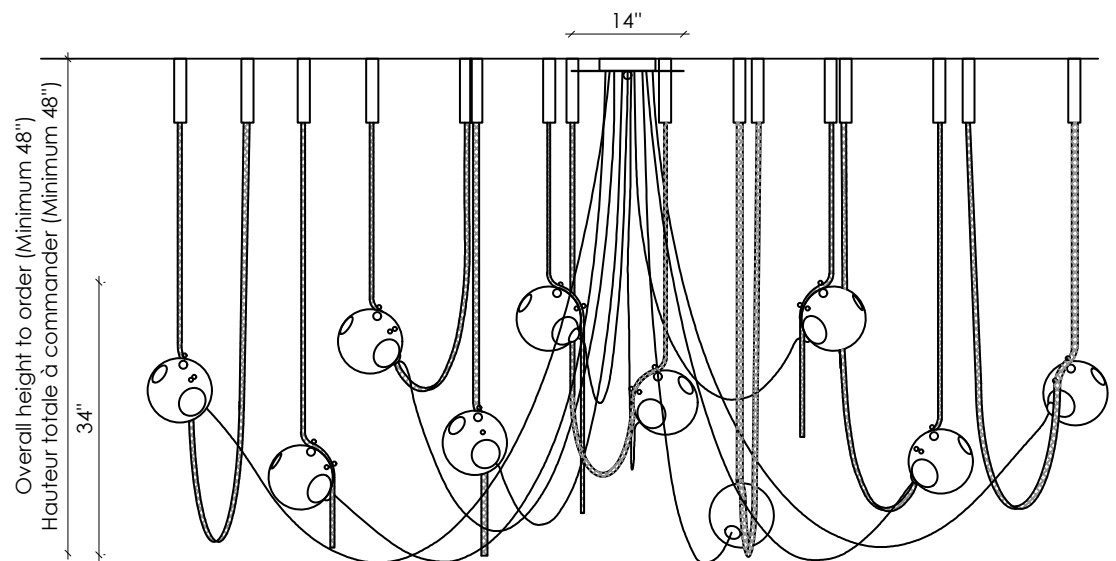
FRONT VIEW VUE DE FACE
