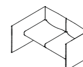
DEL2-S/W-IND-R/L* W 1450 D 1115 / 1190 H 740 S 440
