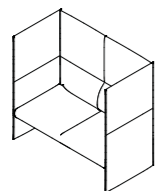
DHL2 W 1450 D 740 H 1300 S 440
