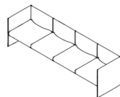
DL4-IND W 2770 D 740 H 740 S 440
