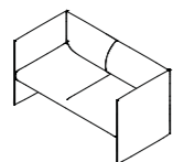
DL2 W 1450 D 740 H 740 S 440
