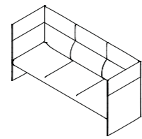
DML3 W 2110 D 740 H 1020 S 440
